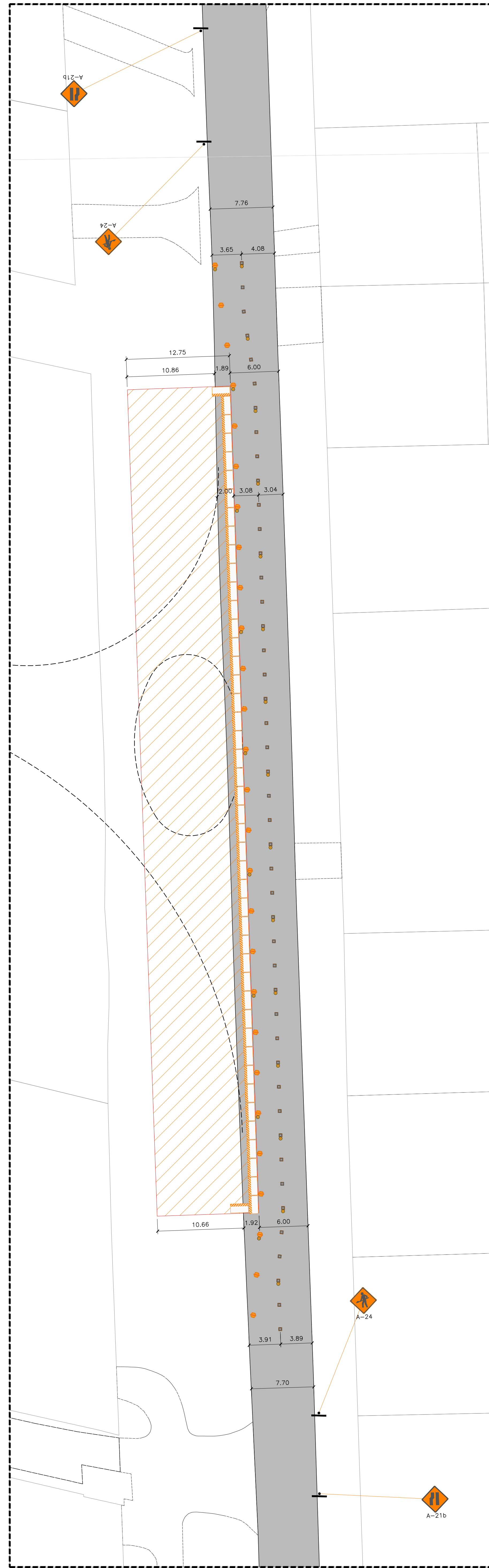
AMPLIAÇÃO - INTERSEÇÃO RUA 1 ESCALA: 1:200
